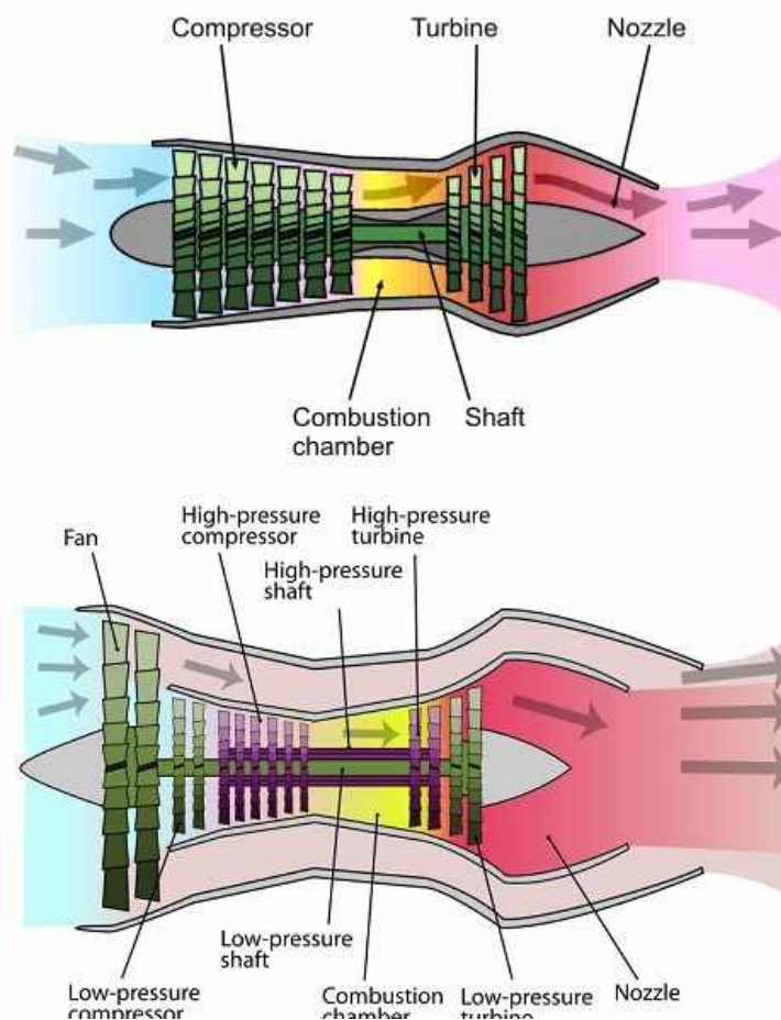
تصویر گرافیکی از موتور توربوجت (بالا) و توربوفن (پائین)
