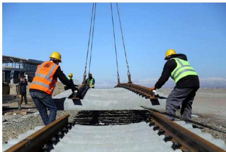
ریل گذاری قطعه رشت، انزلی، آستارا آخرین پازل کریدور شمال - جنوب
