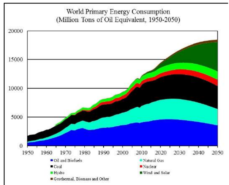
تصویر ۴ - روند مصرف نفت و سایر انرژی ها تا سال ۲۰۵۰
